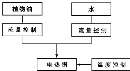
图 2 油烟发生装置示意图
